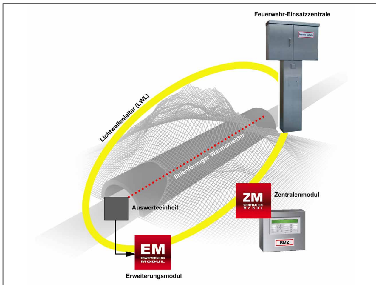
Übersichtsschema Tunnel
